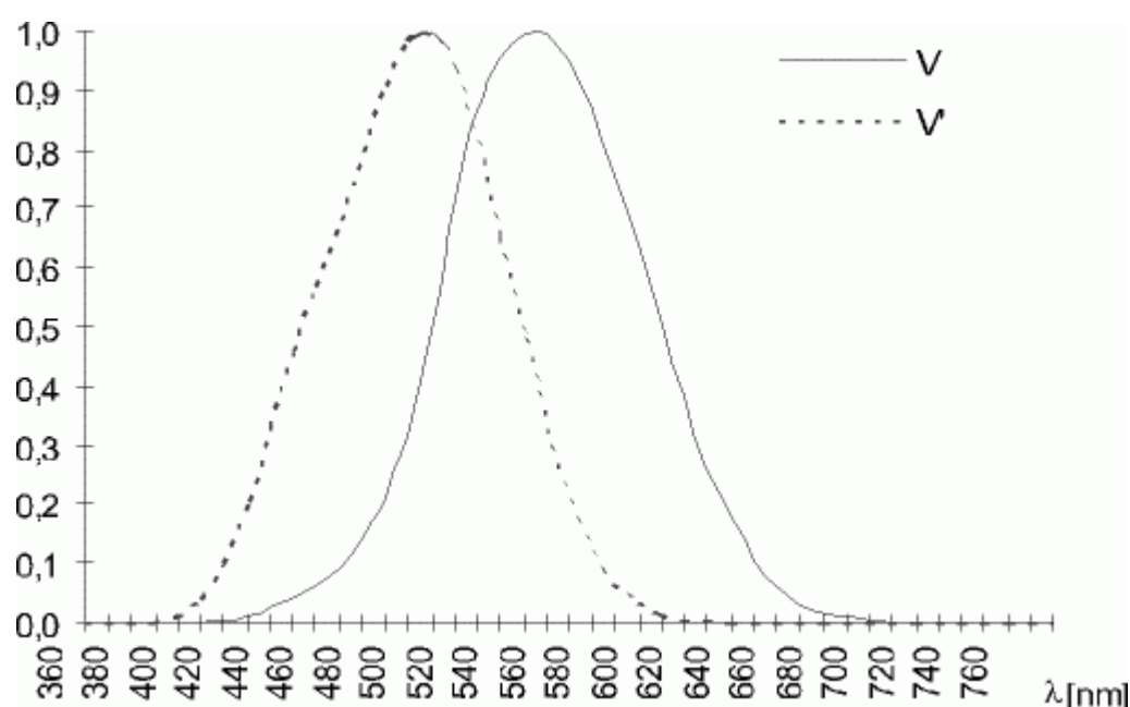
Rys.1 Rozkłady widmowe względnych skuteczności fotopowej: V(\lambda) i skotopowej: V'(\lambda)
